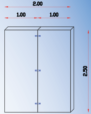
Fixation avec un fer plat acier Hauteur = 2,50
