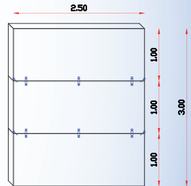
Fixation avec un fer plat acier Hauteur = 3,00
